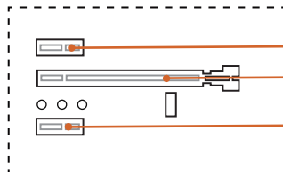
图2-4 PCI扩展插槽
