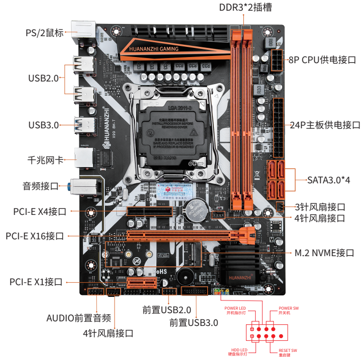
图1-1 X99-8M-T 主板图解
